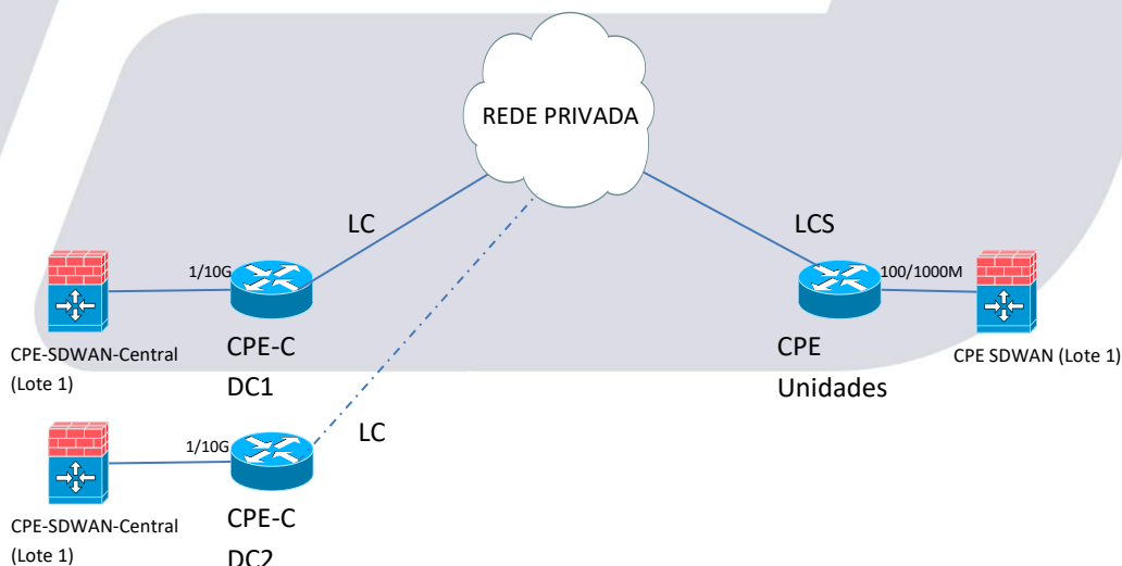
Topologia Lote 2
